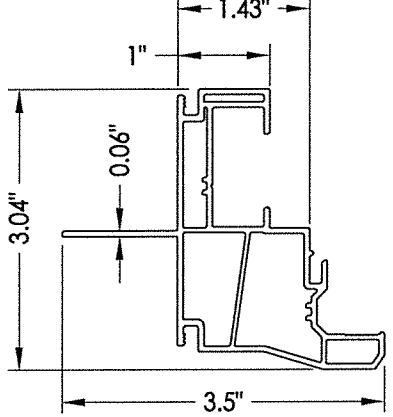
3 FRAME JAMB
